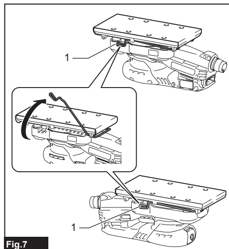
► 1. Levier de serrage
